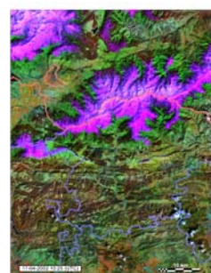
Monitorització mitjançant teledetecció de l'acumulació de neu.
